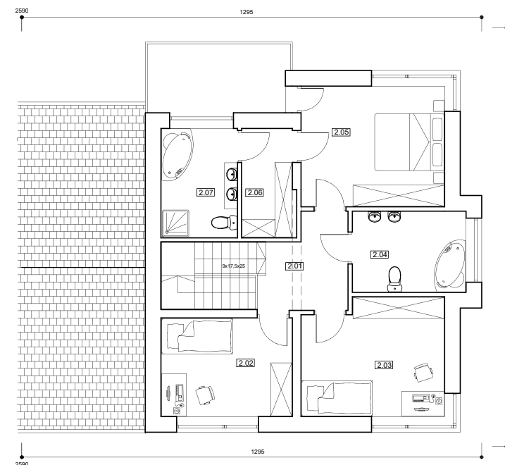
Rzut piętra lokalu A
