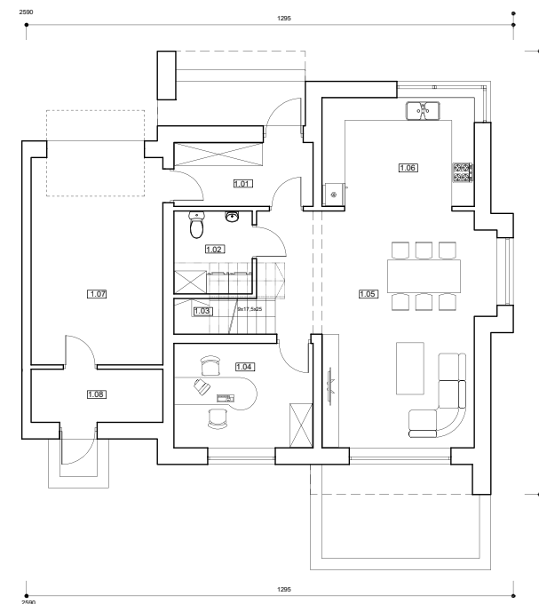
Rzut parteru lokalu A
